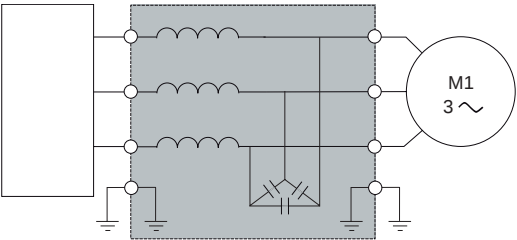
Синусный фильтр
